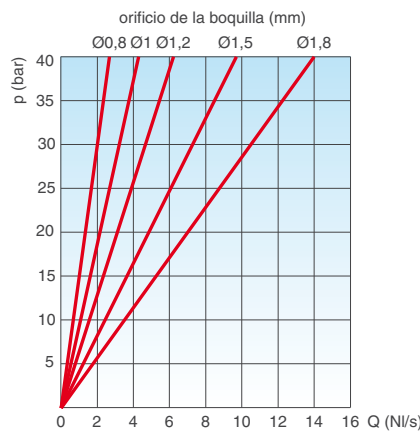
PURGA DE AIRE BAJO PRESIÓN
